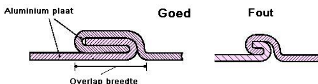
figuur 11 De felsverbinding: links goed, rechts fout
