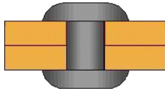
figuur 12 Klinkverbinding
