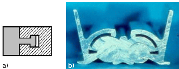
figuur 10 a) Eenvoudige profieldoorsnede waarmee een vaste vormverbinding wordt gevormd; b) Profieldoorsnede waarmee een scharnierende vormverbinding wordt gevormd
