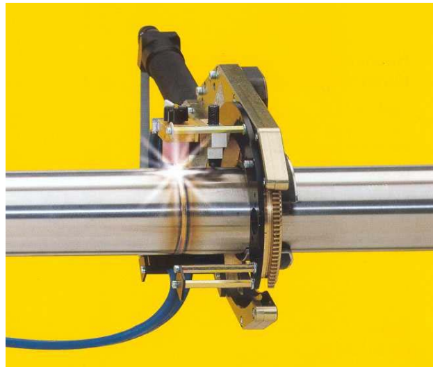
figuur 1 Het gemechaniseerd TIG-lassen van een pijp/pijpverbinding
