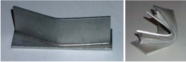
figuur 2 Vlamgesoldeerde verbinding in aluminium (stompe verbinding in aluminium - EN AW-1050). Na het solderen (links) en na het vervormen van het product (rechts)
